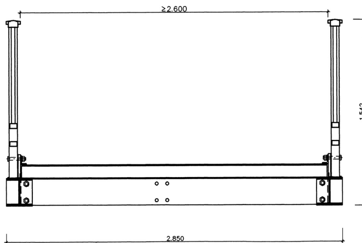
FB-10/2,5 Querschnitt
