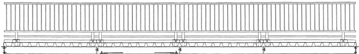
FB-10/2,5 Längsschnitt
