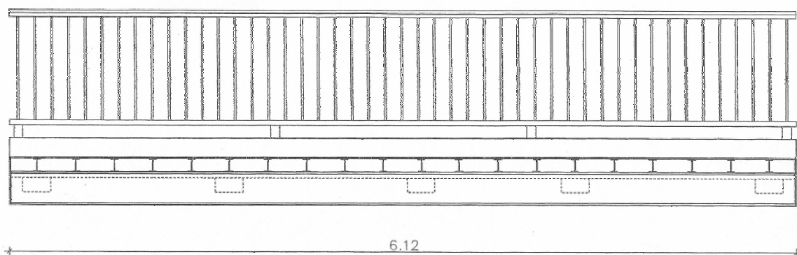
Längsschnitt
