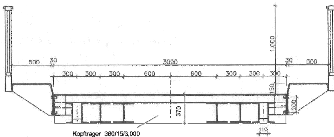
Querschnitt
